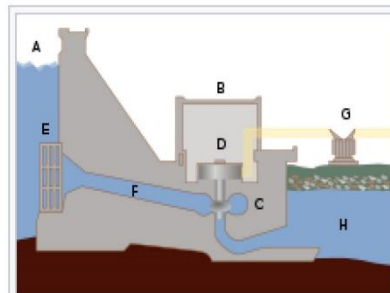
Schéma en coupe d'un barrage hydroélectrique. A : réservoir, B : centrale électrique, C : turbine, D : générateur, E : vanne, F : conduite forcée, G : lignes haute tension, H : rivière
