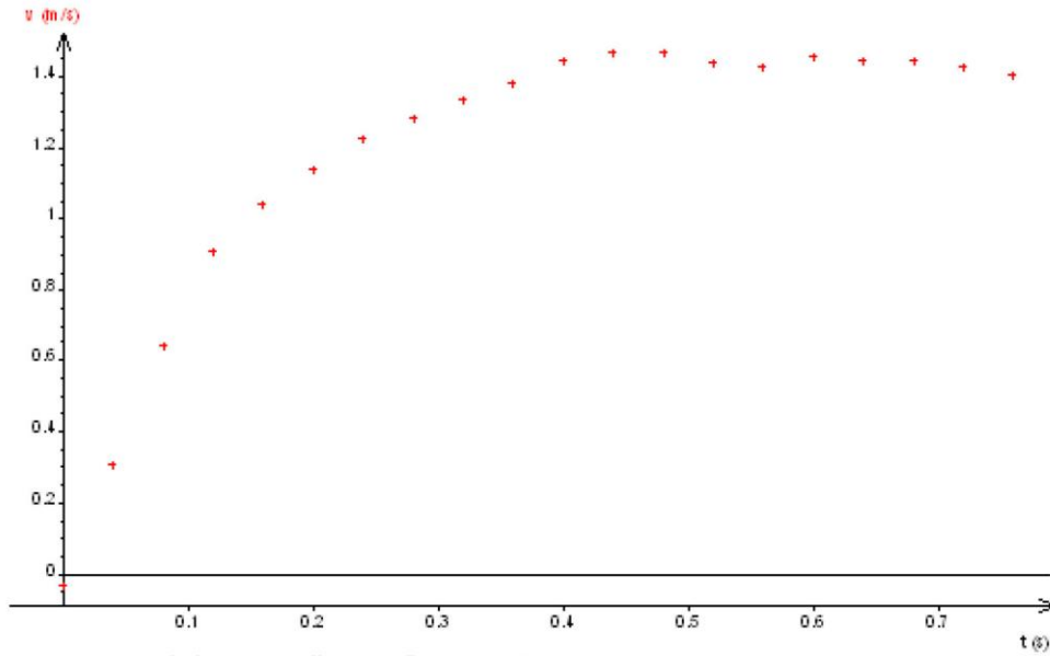
منحنى تغير سرعة مركز قصور الكرية خلال سقوطها في سائل الغليسيرول مخفف
